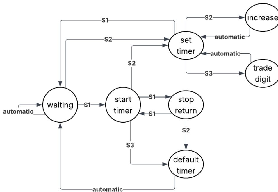
Figura 1 - digrama de máquina de estados do temporizador
