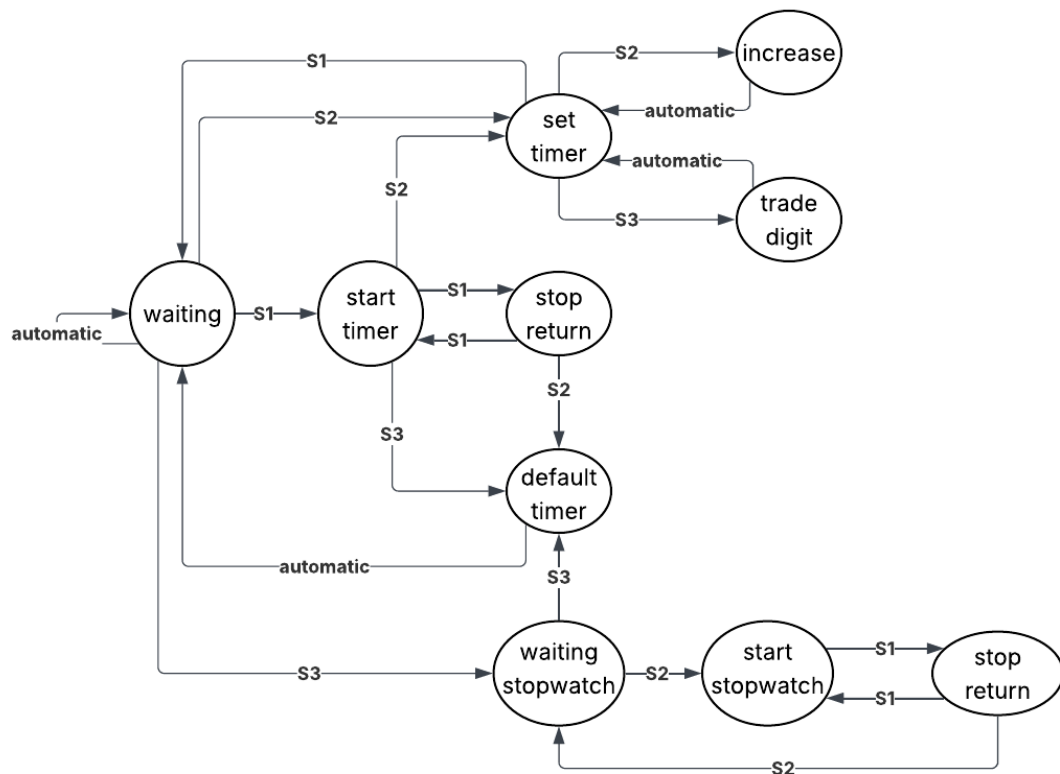
Figura 2 - Máquina de estados do cronometro
